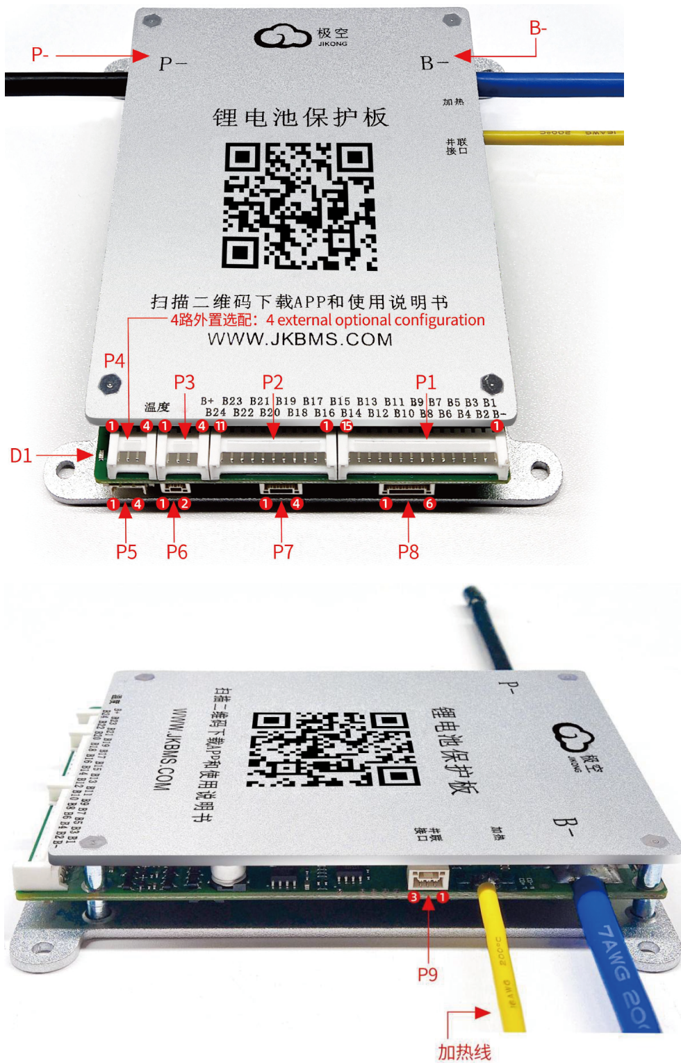
JK-BD4AxxS-6P/8P 连接器示意图
