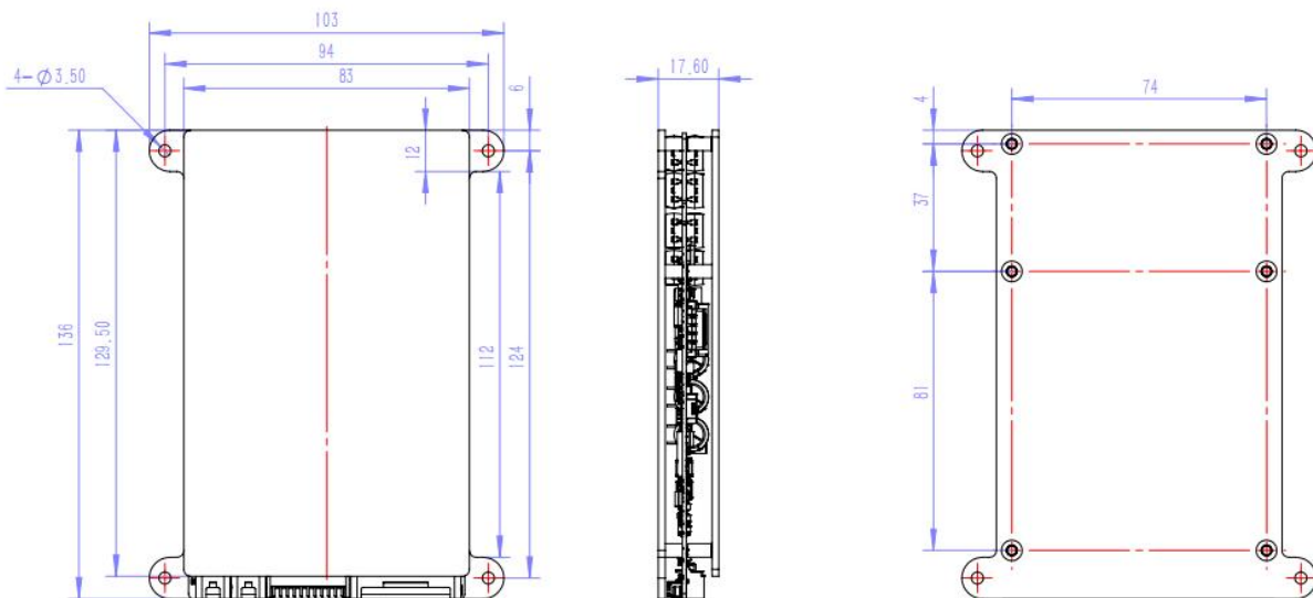
JK-BD4AxxS-6P/8P 外形尺寸
